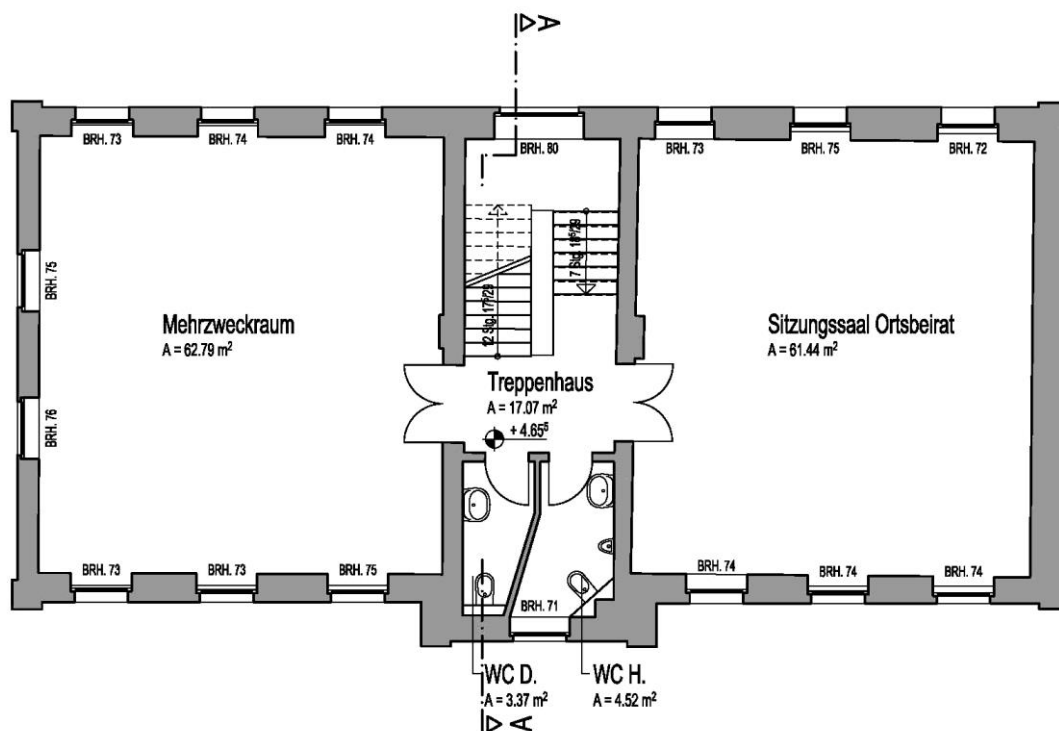
Grundriss Obergeschoss
