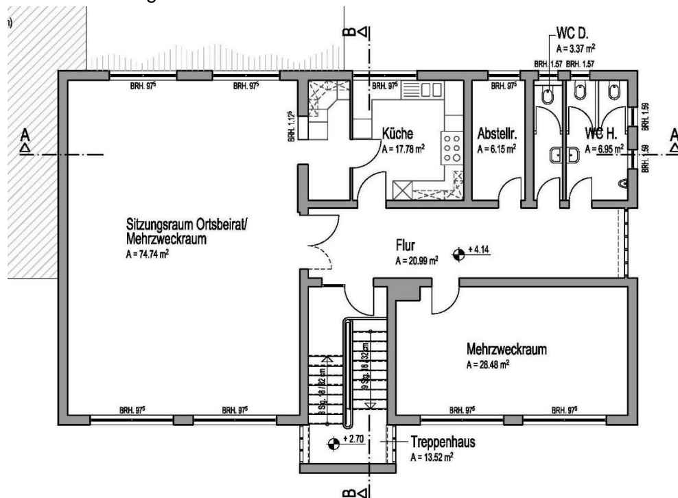
Grundriss Obergeschoss
