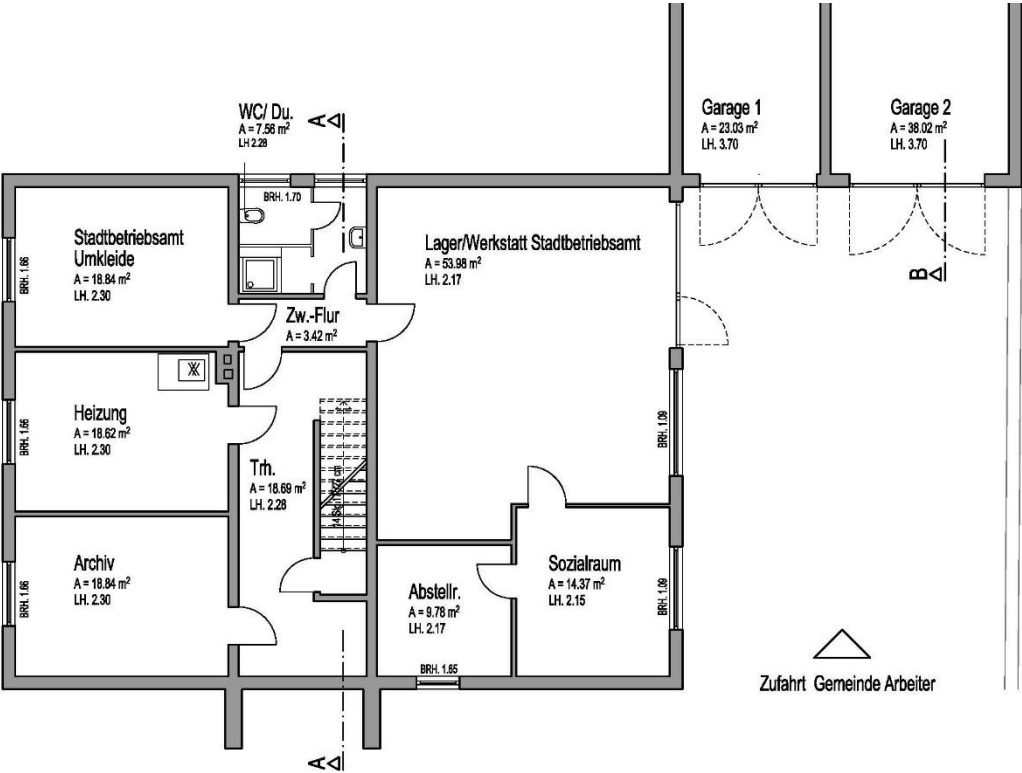
Grundriss Untergeschoss
