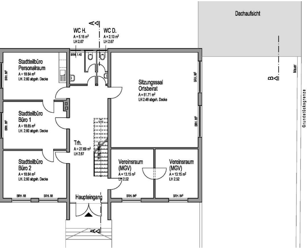
Grundriss Erdgeschoss
